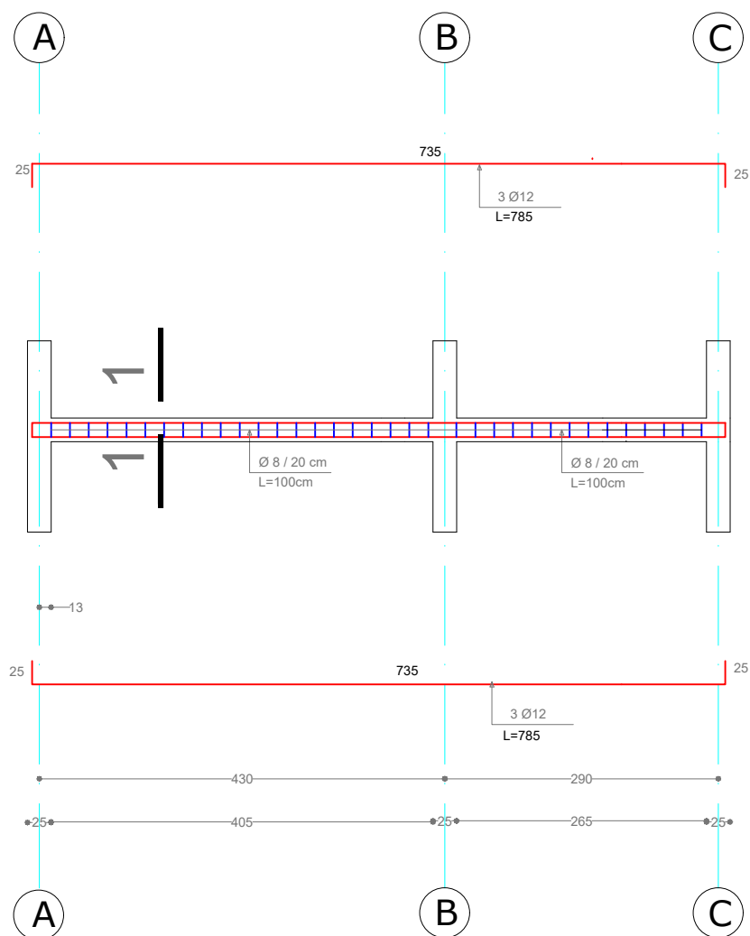
ARMIMI I BREZIT NE AKSIN 2-2
