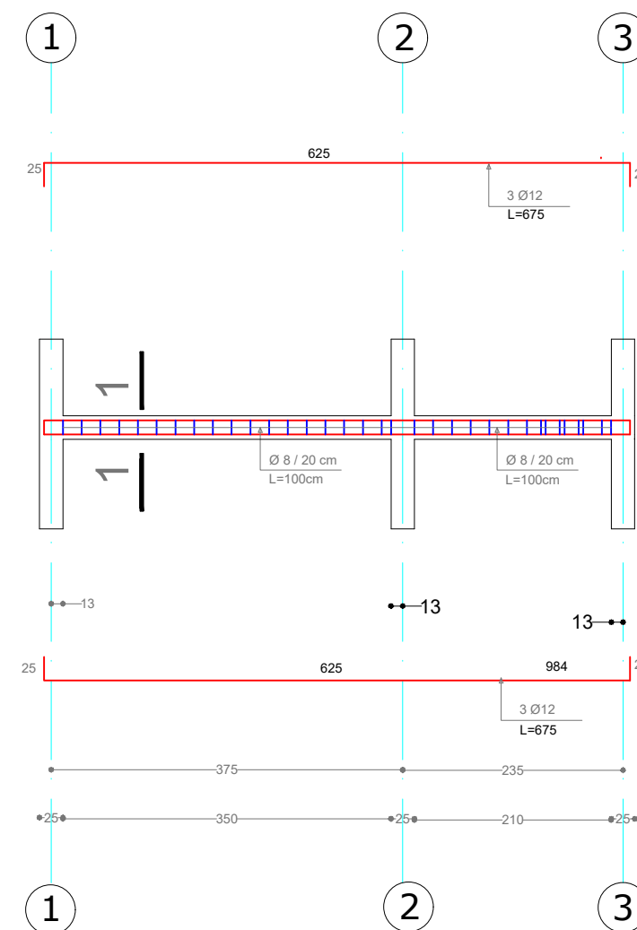
ARMIMI I BREZIT NE AKSIN B-B
